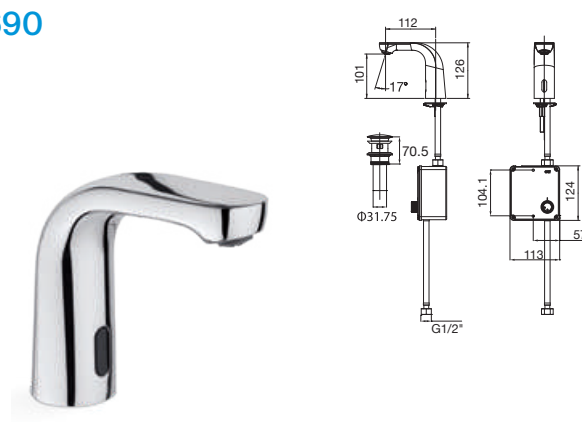
L20 感應面盆單冷龍頭 (交流電 AC) Z5A5709C4N
