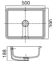
Sofia 枱底盆 A3270YD000
