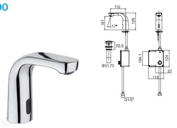
L20 感應面盆單冷龍頭 (電池DC) Z5A5609C4N
