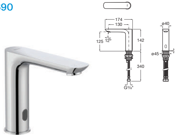
CALA-E 感應面盆單冷龍頭 (交流電 AC) A5A576EC0G
