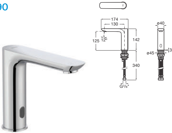
CALA-E 感應面盆單冷龍頭 (電池DC) A5A566EC0G
