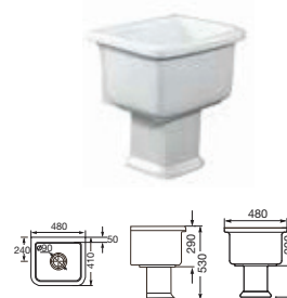
HAMITO-S 拖把池 / 拖把池企柱 A371455000 $1,860 480 410 290 mm A371456000 企柱 $560 180 220 240 mm
