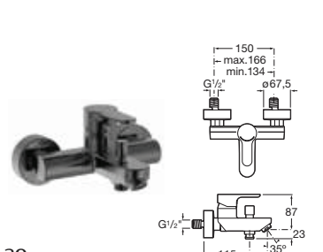
L20 浴缸龍頭
