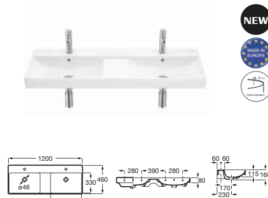
ONA 掛牆盆 (雙盆)
