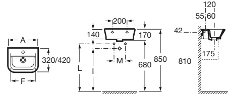
THE GAP 小型面盆 (掛牆·枱上盆兩用)
