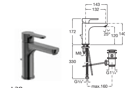
L20 面盆龍頭
