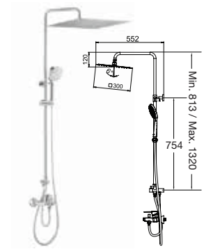
MITOS 方形雨淋淋浴柱 (300x300mm) (可調校高度)
