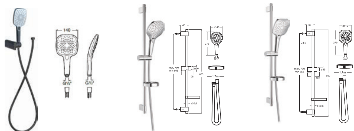
L20 / ATLAS 花灑套裝
