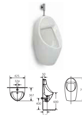
EURET 小便器 (頂入水) Z35945H000 $4,540 425 367 797 mm
