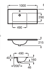
DEBBA 一體式面盆 (左翼)
