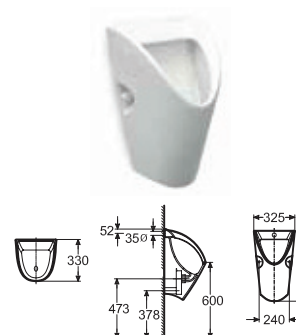
CHIC 小便器 (後入水) Z35945J000 $2,480 325 330 558 mm
