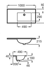
DEBBA 一體式面盆 (左翼)
